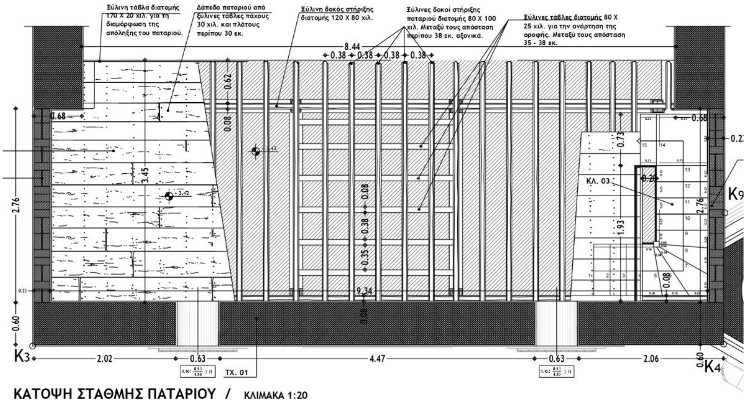
Σχέδιο 16 – Κάτοψη στάθμης παταριού/γυναικωνίτη (λεπτομέρειες δαπέδου), στάθμη: 3.43μ
