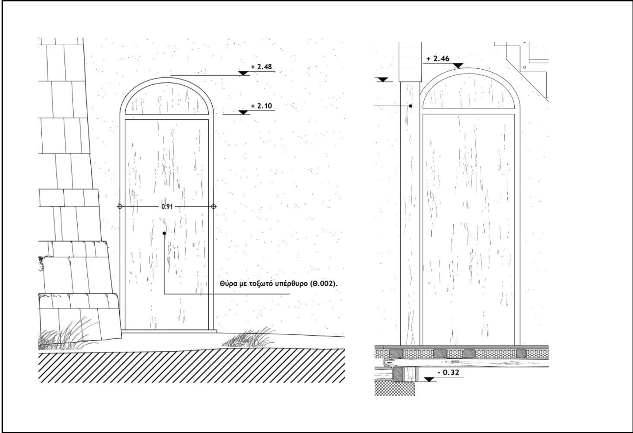
Σχέδιο 9 – Κούφωμα εισόδου (θ.002) στη βορειοδυτική πλευρά του κτιρίου (όψεις εξωτερικά και εσωτερικά)
