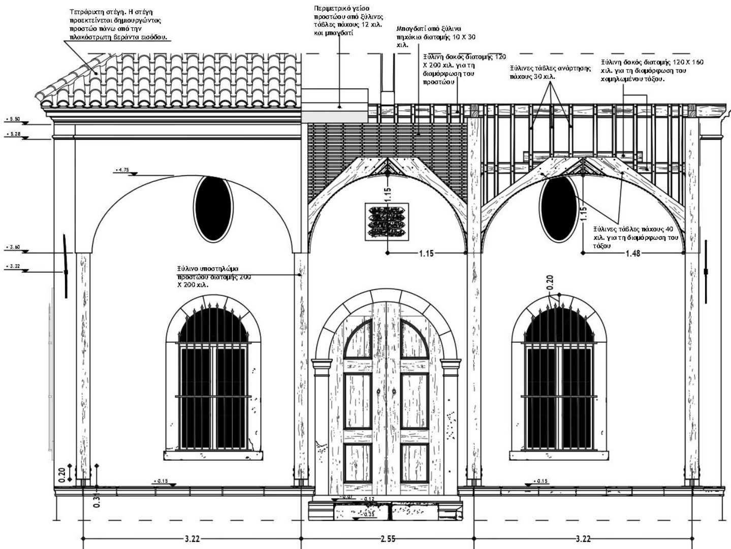
Σχέδιο 22 – Βόρεια όψη προστώου
