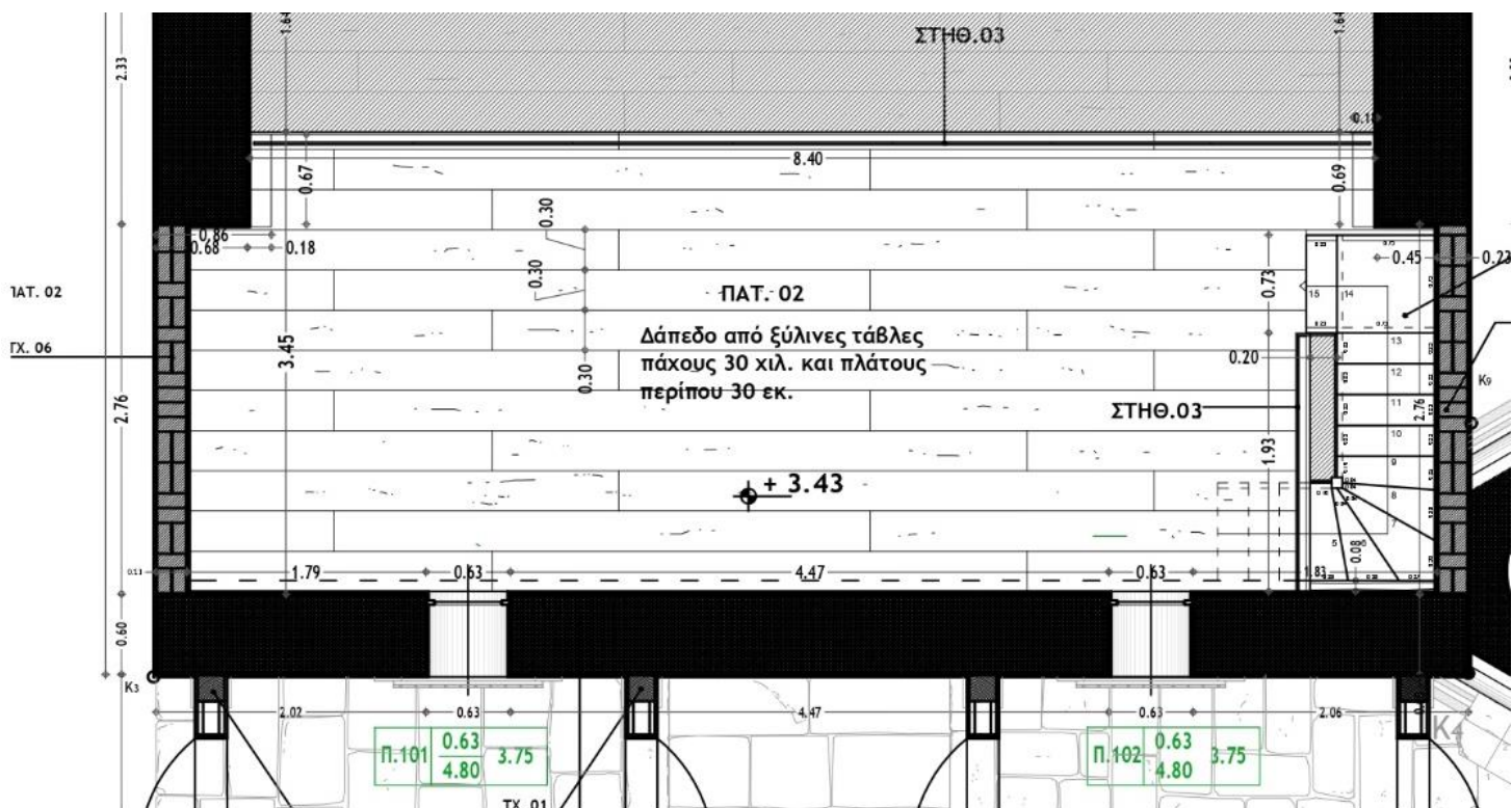
Σχέδιο 17 – Κάτοψη στάθμης παταριού/ γυναικωνίτη, στάθμη: 3.43μ
