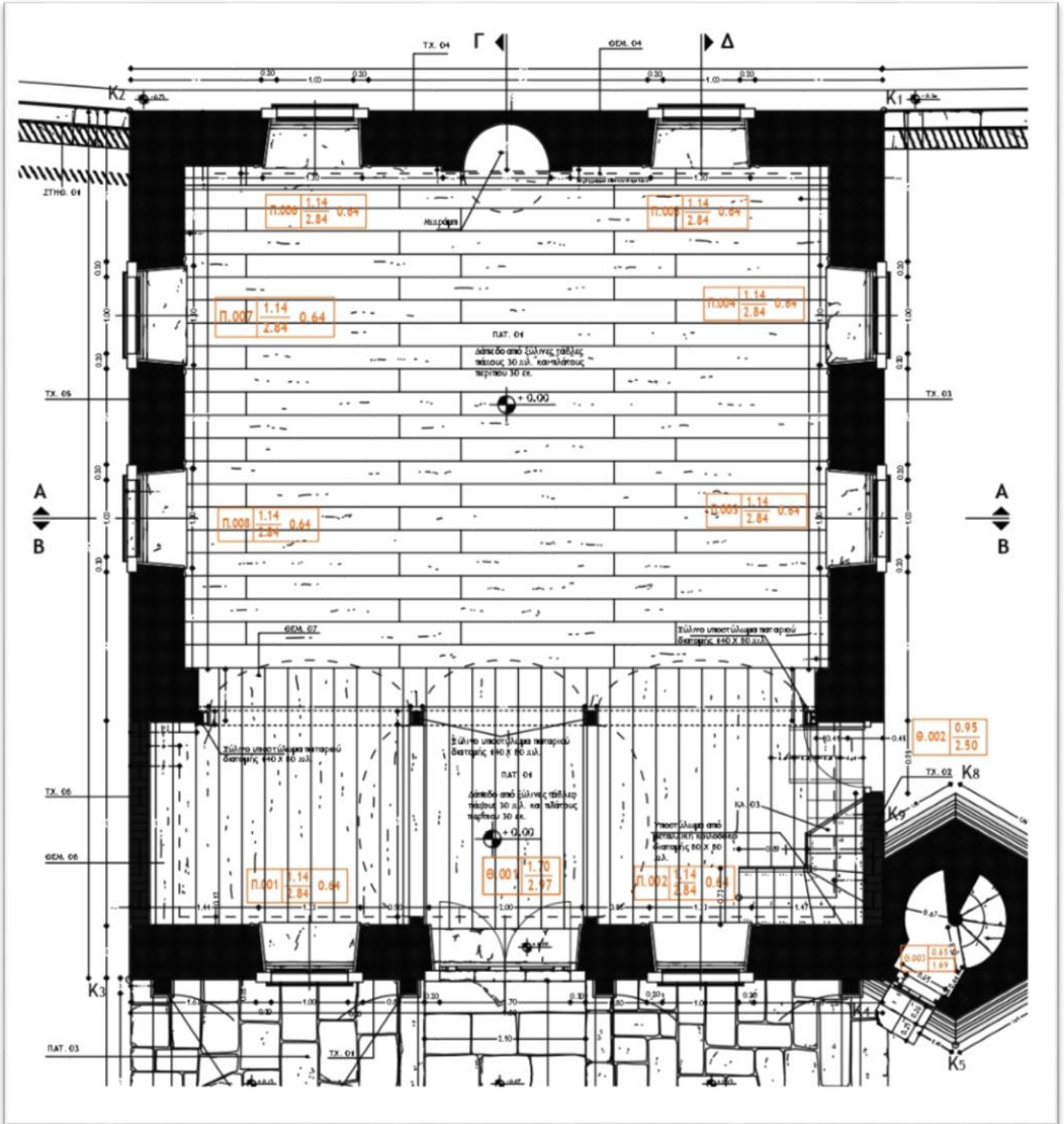
Σχέδιο 1 - Κάτοψη ισογείου (Κουφώματα-θύρες)
