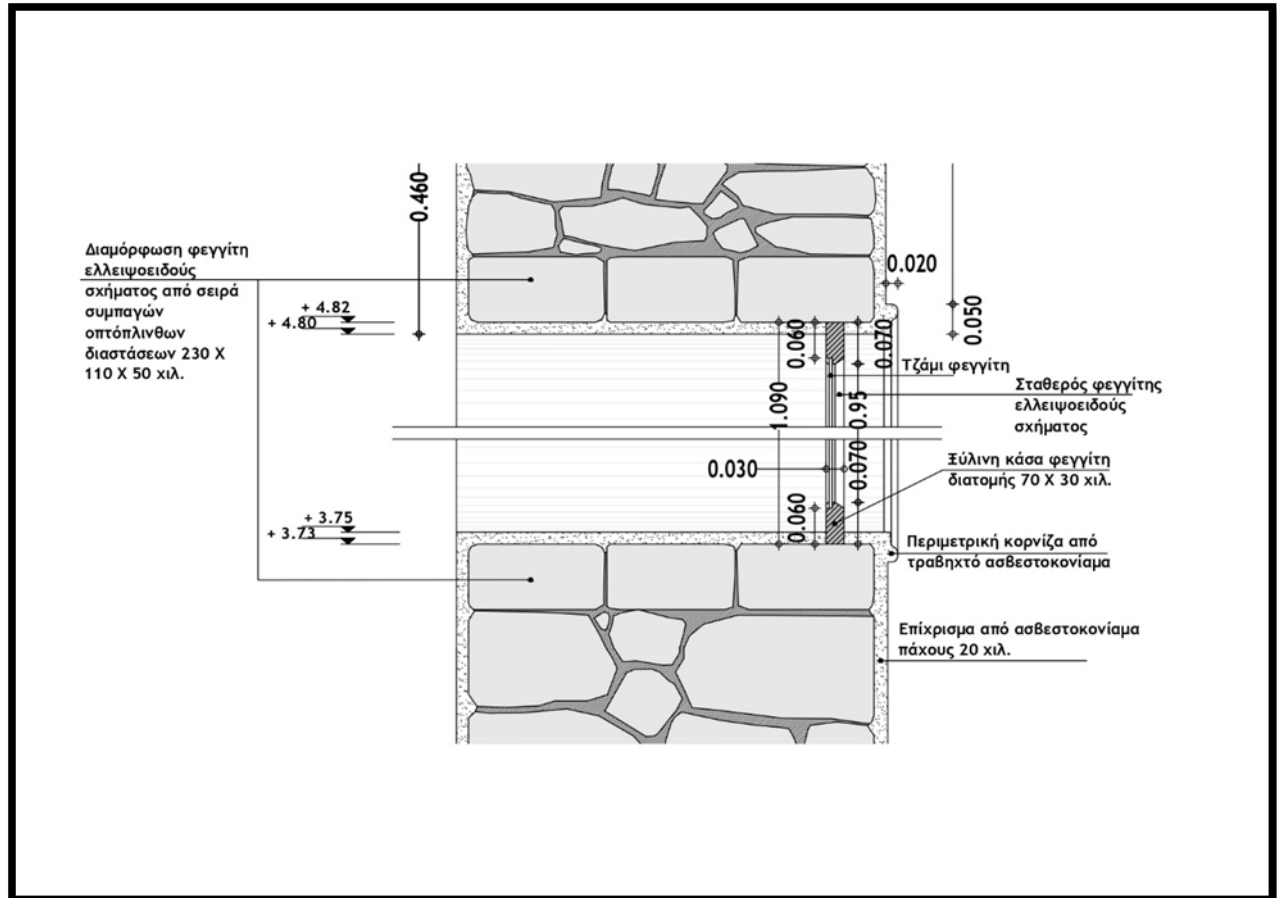
Σχέδιο 5 – Φεγγίτης : κατακόρυφη κατασκευαστική τομή (Π.101-Π.108)
