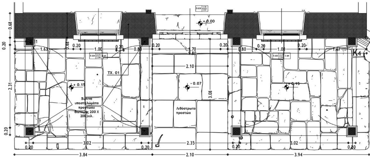
Σχέδιο 21 – Κάτοψη στάθμης ισόγειου προστώου
