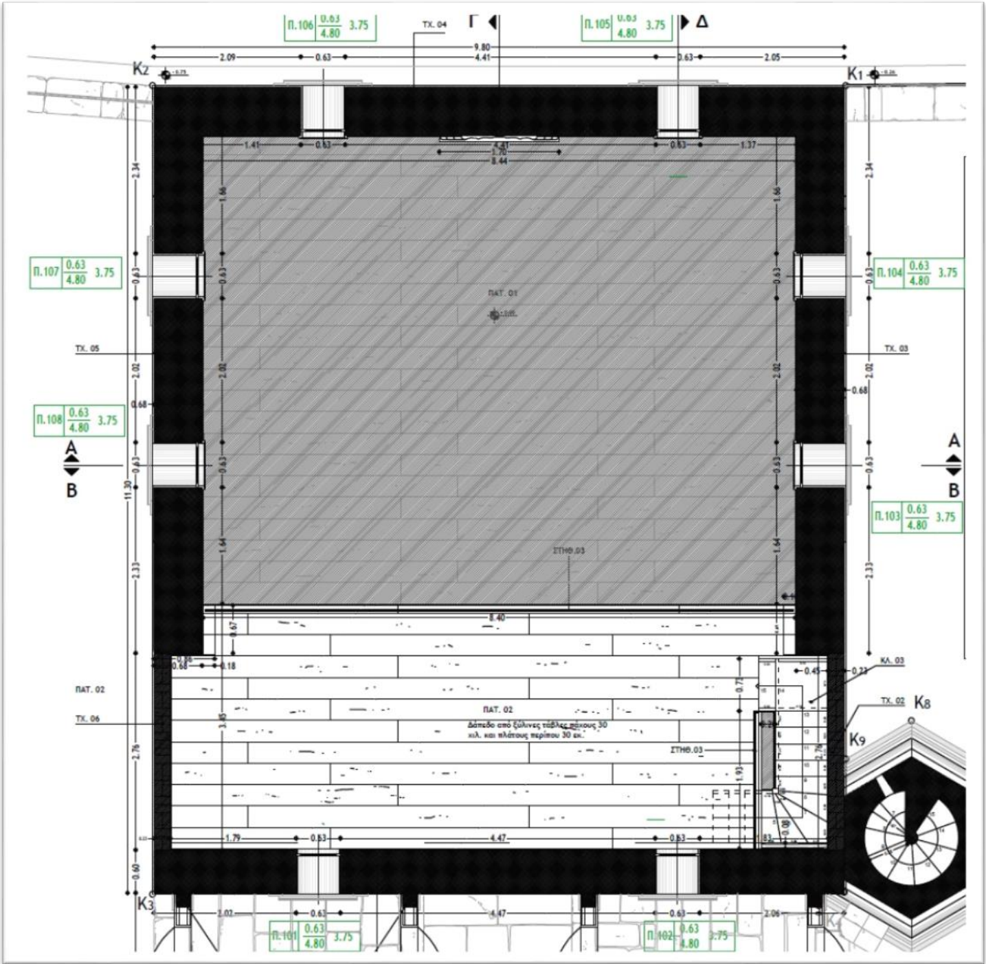
Σχέδιο 2 - Κάτοψη παταριού – γυναικωνίτη (Φεγγίτες)
