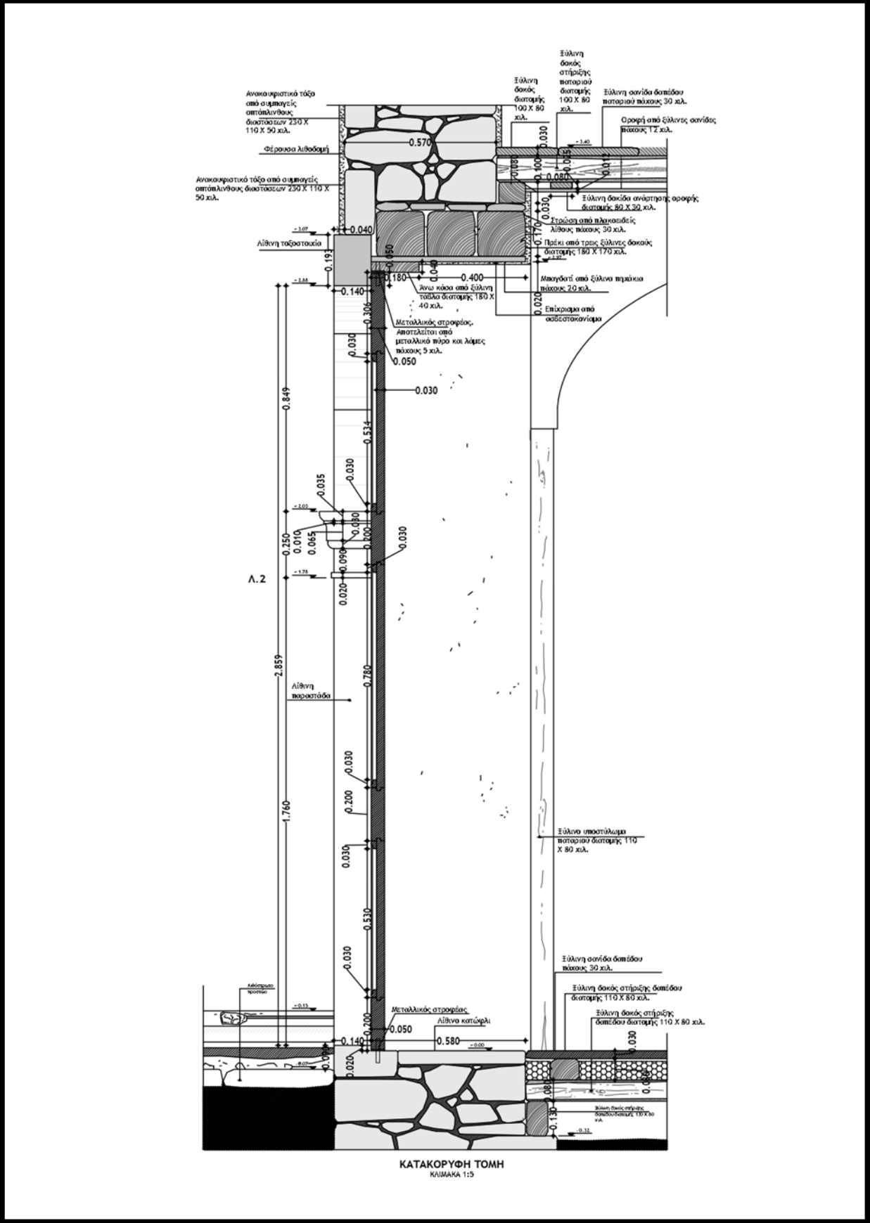
Σχέδιο 6 – Κούφωμα κεντρικής εισόδου (0.001) – Κατακόρυφη τομή
